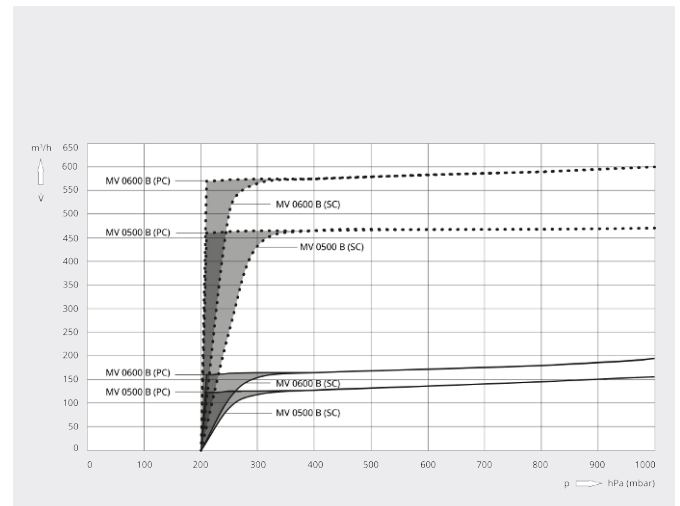
抽氣速率
