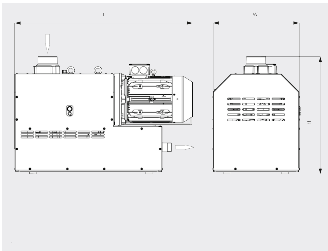
尺寸圖
